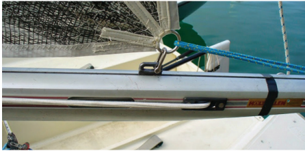
L'élastique de rappel rentre dans la bôme pour faire 3 allers retours.
